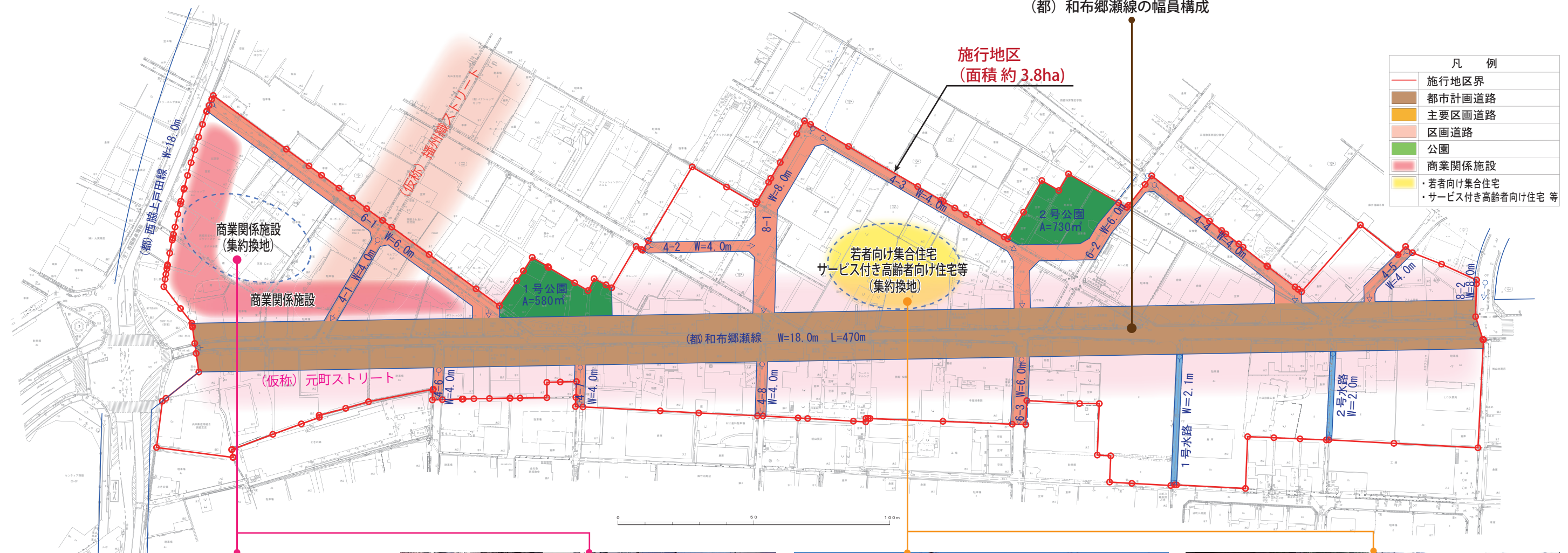
(都) 和布郷瀬線の幅員構成
