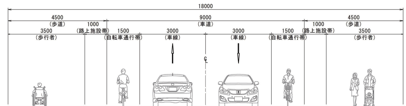
(都) 和布郷瀬線の幅員構成
