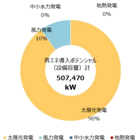
図5-9 【再掲】再生可能エネルギーの導入ポテンシャル（出典：環境省 自治体排出量カルテ/西脇市）
