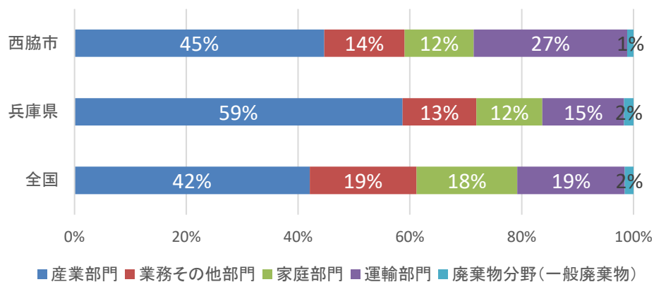
図2-28 部門別CO 2 排出量構成比の比較（出典：環境省）
