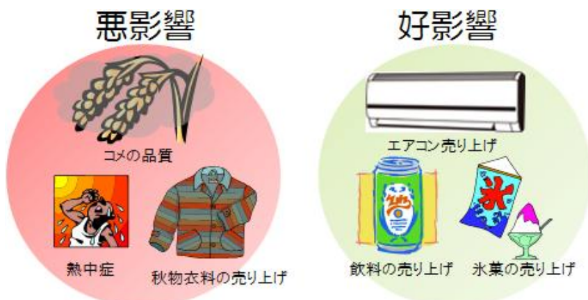
図5-4 平成22(2010)年夏の猛暑の影響(出典:気象庁)
