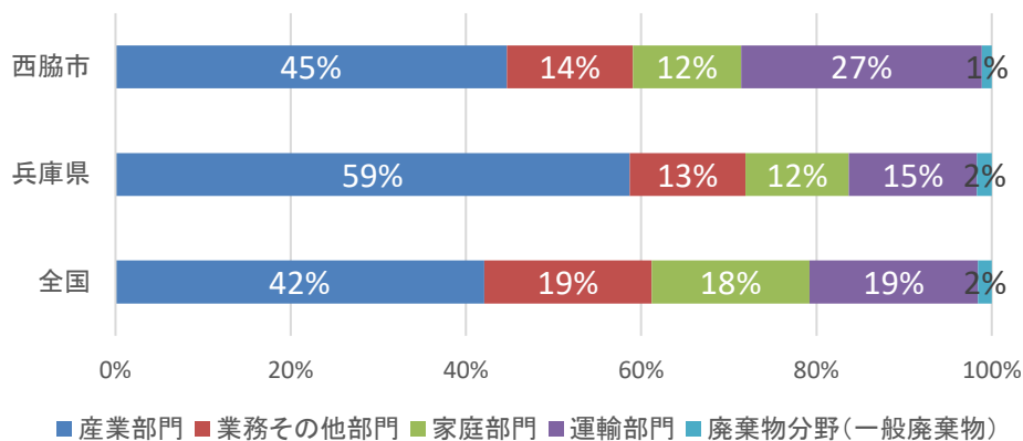
図5-7 【再掲】部門別CO 2 排出量構成比の比較 (出典：環境省 自治体排出量カルテ/西脇市)
