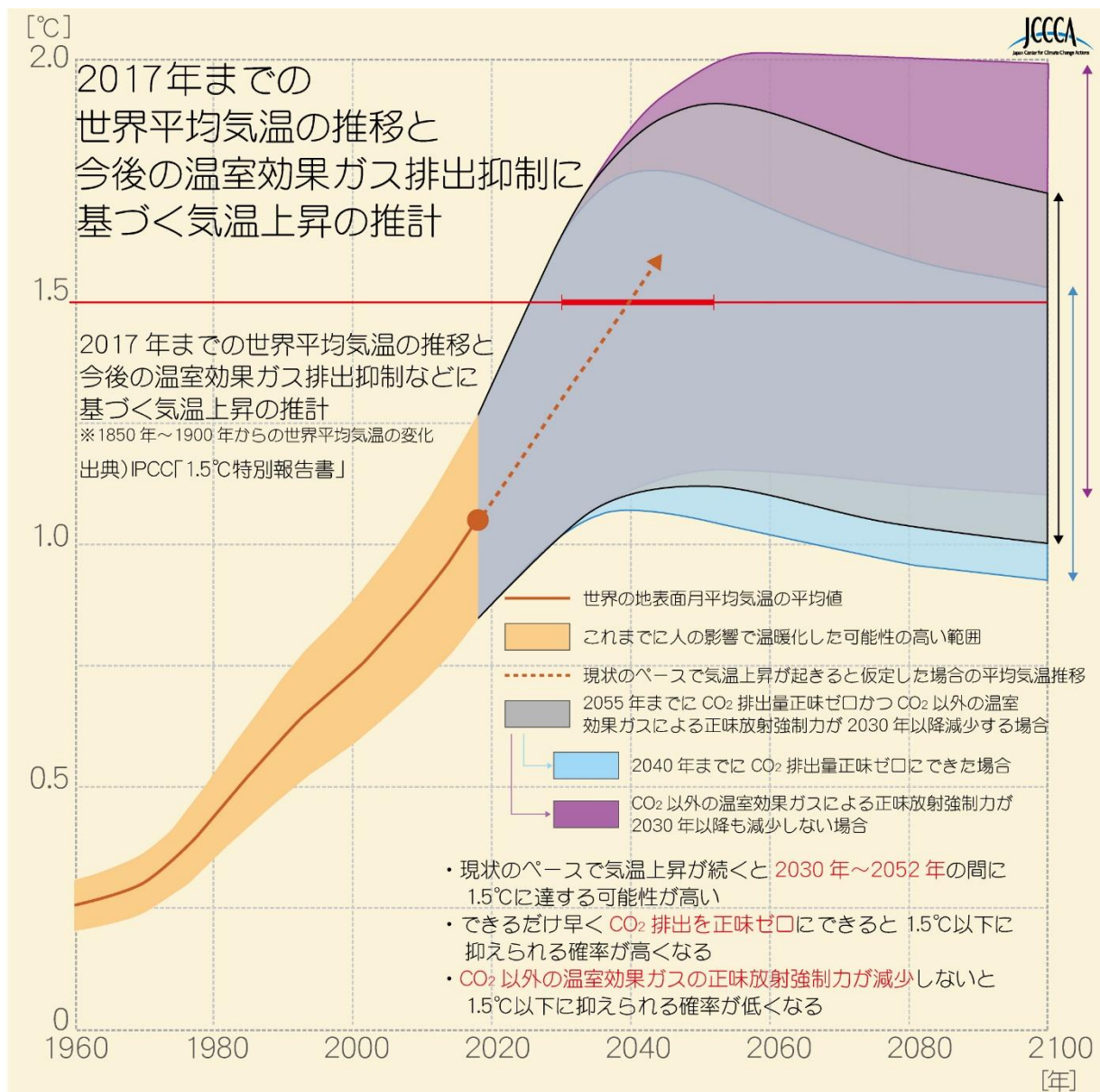
図5-3 2017年までの世界平均気温の推移と今後の温室効果ガス排出抑制に基づく気温上昇の推計 (出典：「1.5℃特別報告書」IPCC)
