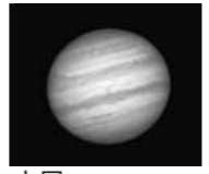
木星
