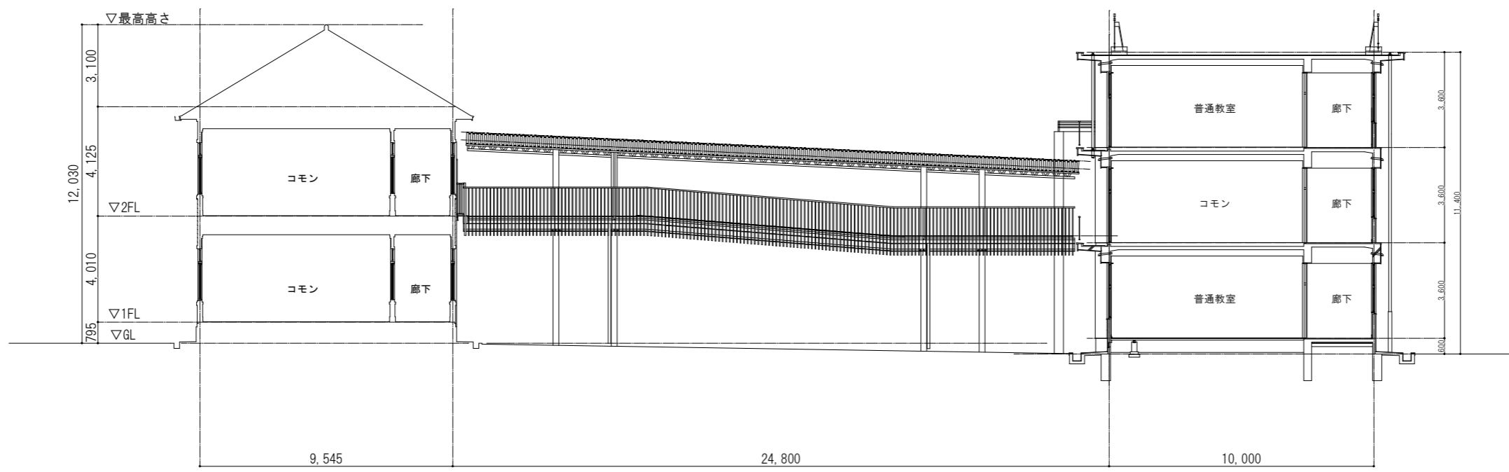
2階渡り廊下C 東立面図
