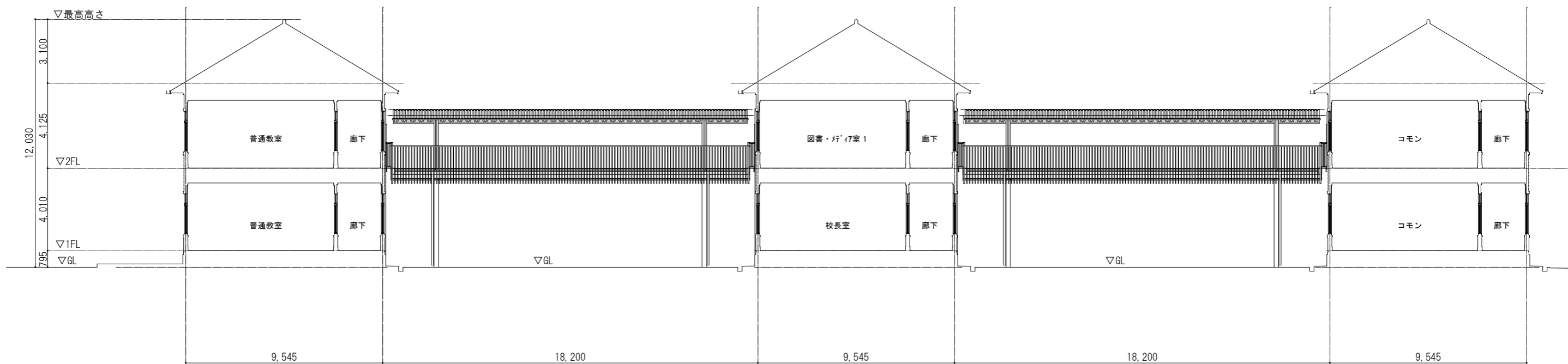
2階渡り廊下A 東立面図
