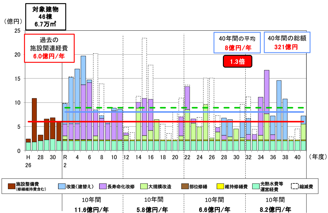
図表 6.3.1 維持・更新コスト（長寿命化型）
