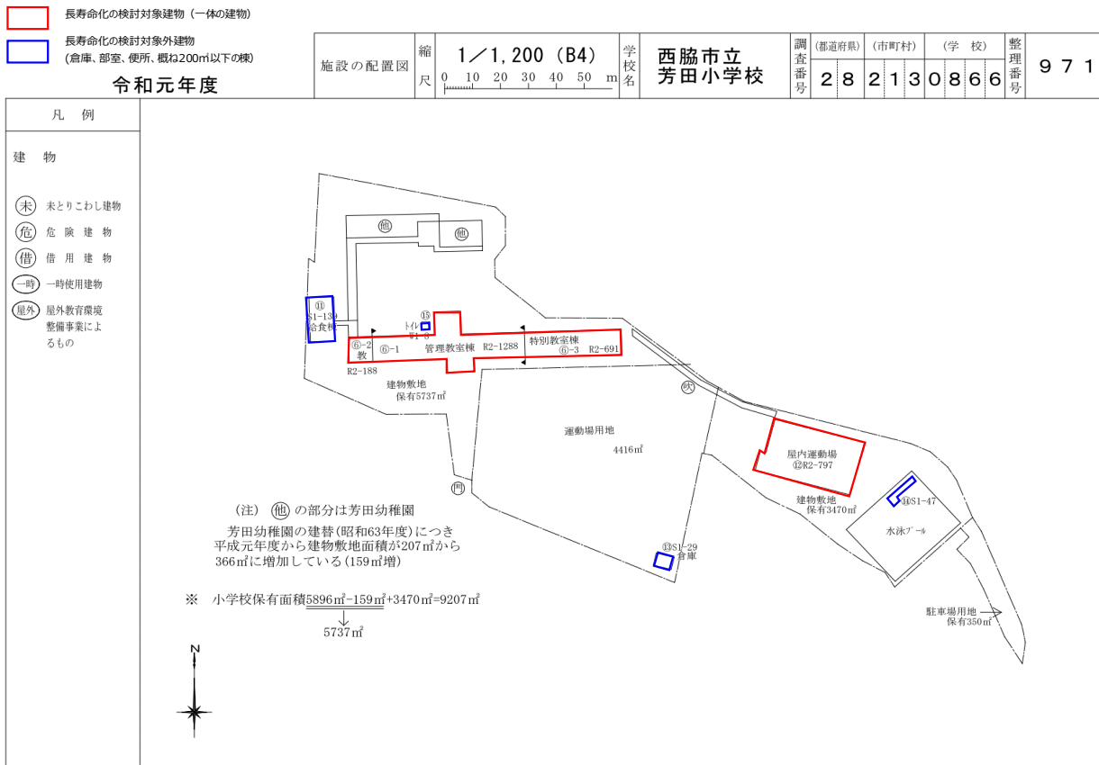
図表 1.4.10 芳田小学校（平面図）
