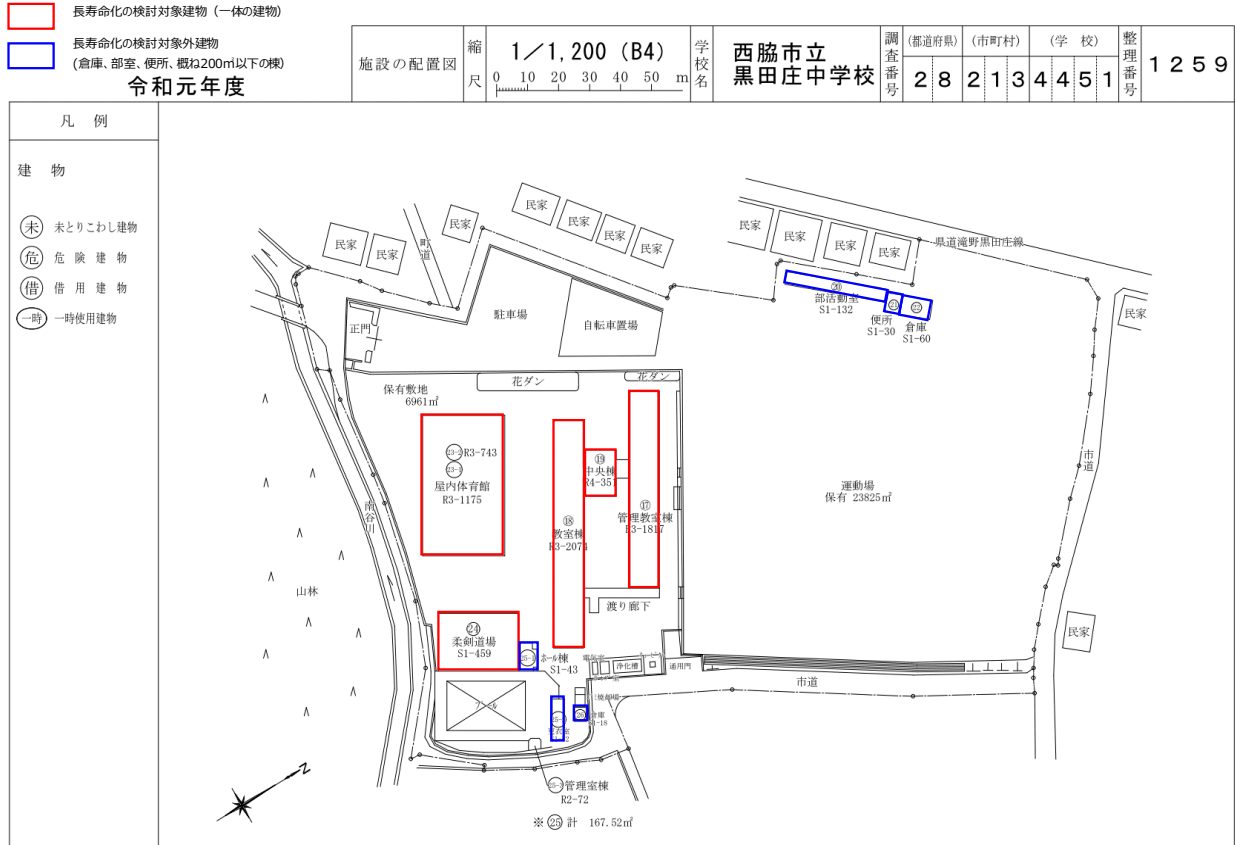
図表 1.4.16 黒田庄中学校（平面図）
