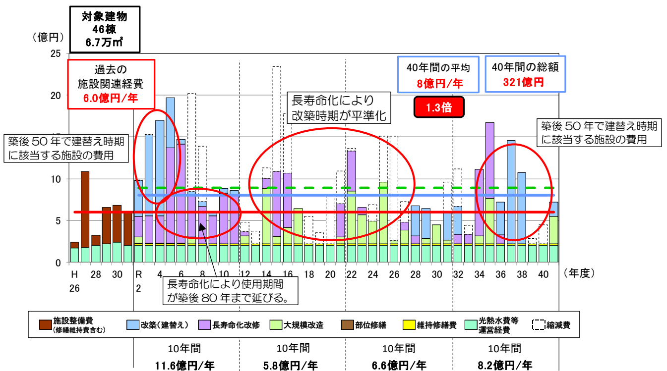
図表 6.3.6 維持・更新コスト（長寿命化型）※再掲
